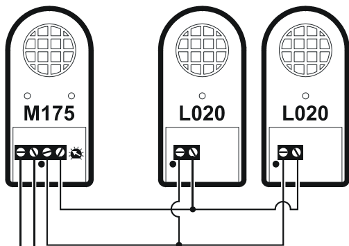
Anschlussmöglichkeit für 2 Zusatzlautsprecher L020 Possibility to connect 2 additional loudspeakers L020
